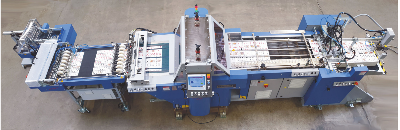
Automatische Spielkartenproduktionsanlage, bestehend aus BOGRAMA Stanzmaschine BSR 550 Servo und Spielkartenauslage ACC 550 HS
